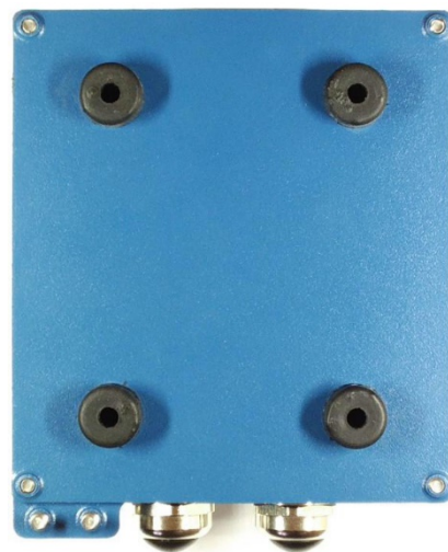
Abmessungen Befestigungslöcher
