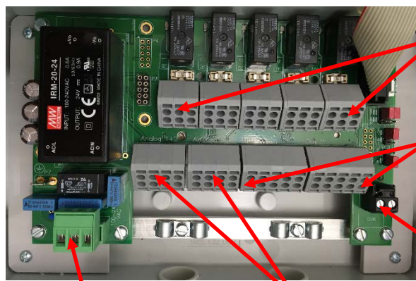
Einspeisung 230 VAC
